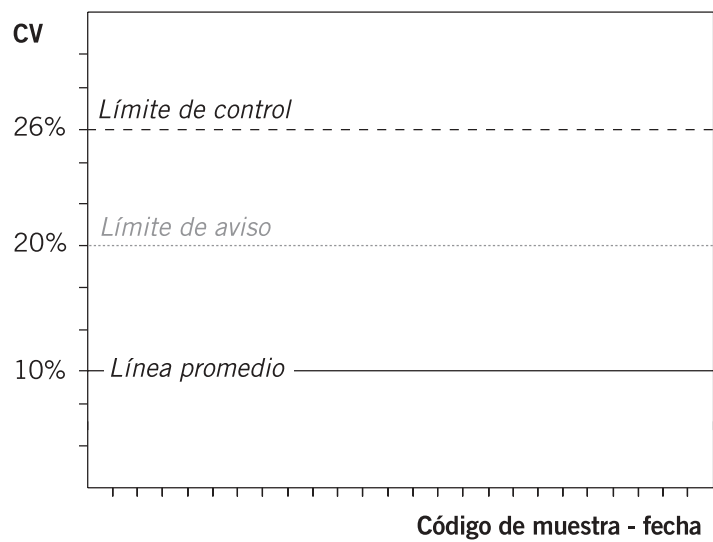
Figura 1: Gráfico de control elaborado para un nivel de precisión del 10%
